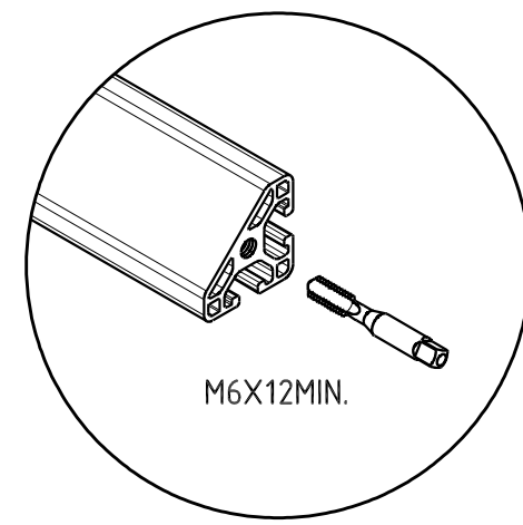
DETTAGLIO 2 SCALA 1:2
