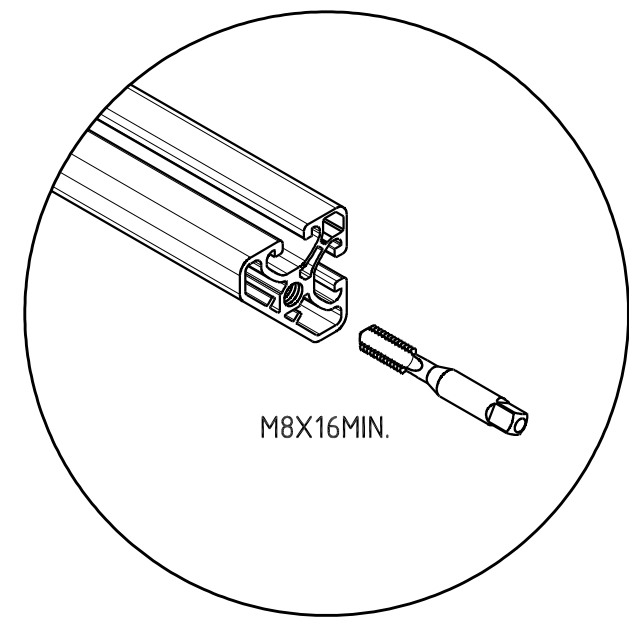
DETTAGLIO 1 SCALA 1:2
